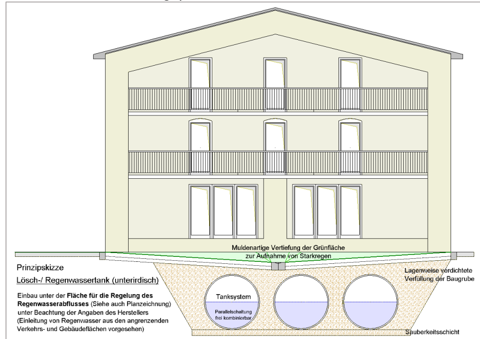
Abbildung 16: Prinzipskizze für den Einbau von Wassertanks
